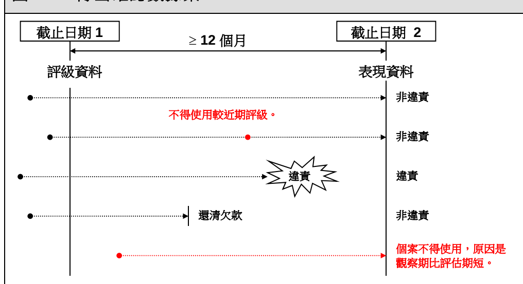
圖 A1. 得出確認數據集
